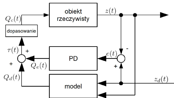
Rys. 2. Schemat blokowy układu sterowania obiektem niedosterowanym Fig. 2. A block diagram of an underactuated system control process.
