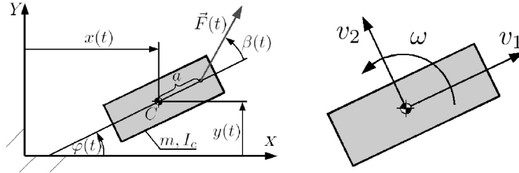
Rys. 1. Model układu niedostereowanego - bryła sterowana siłą niecentralną Globalny układ współrzędnych położenia i lokalne współrzędne prędkości
