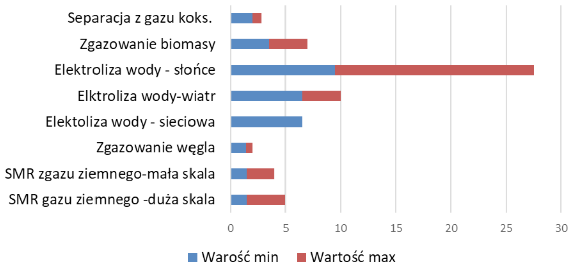
Rys. 3. Szacowane koszty produkcji wodoru w zależności od technologii 1 , USD/kg
