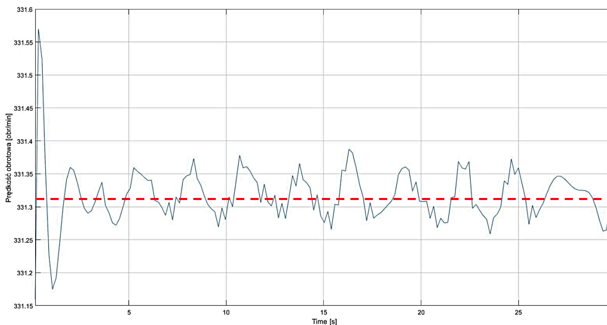
Rys. 13. Wykres chwilowej prędkości obrotowej wałka krzywkowego i jej wartość średnia
