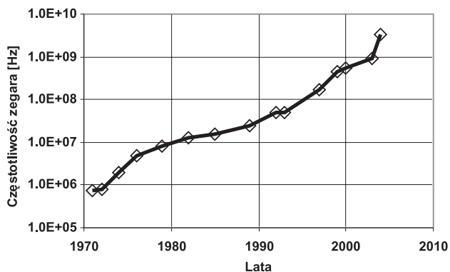
Rys. 7. Zmiana częstotliwości pracy procesorów w funkcji czasu
