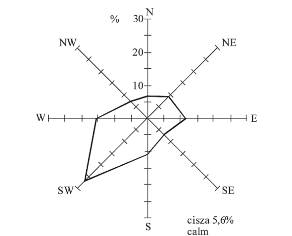
Rys. 6. Procentowy udział poszczególnych kierunków wiatrów towarzyszących opadom atmosferycznym Fig. 6. A percentage distribution of wind directions accompanying atmospheric precipitation
