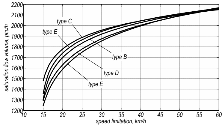
Fig. 2. The dependencies of the saturation flow volume under different types of speed limitation patterns Рис. 2. Зависимости интенсивности потока насыщения при разных типах ограничения скорости
