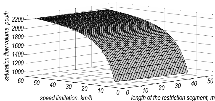
Fig. 3. Dependence of the saturation flow volume on speed limitation and length of the restriction segment Рис. 3. Зависимость интенсивности потока насыщения от ограничения скорости и длины участка ограничения
