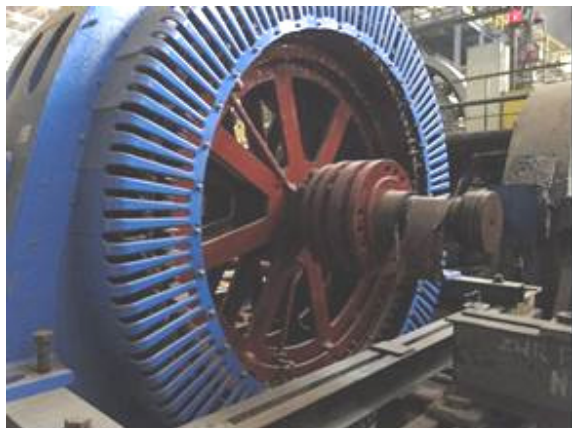
Rys. 1. Widok silnika typu SAS po remoncie
