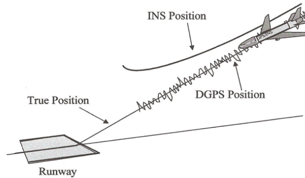
Fig. 5. Position Error Characteristics of the INS and DGPS Rys. 5. Charakterystyki błędu pozycji dla INS i DGPS
