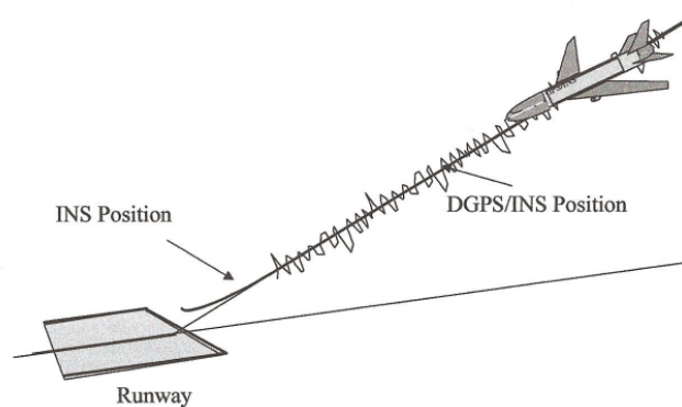
Fig. 6. Position Error Characteristics of the Integrated DGPS/INS Rys. 6. Charakterystyki błędu pozycji zintegrowanego dla DGPS/INS
