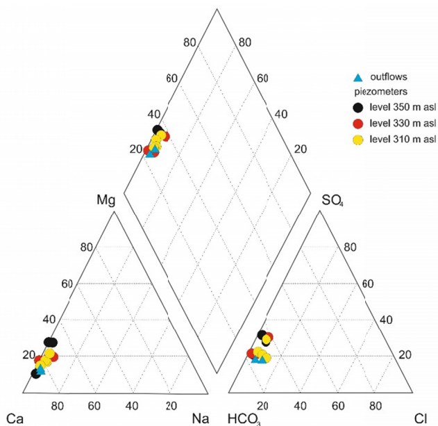
Fig. 7. Piper Diagram
