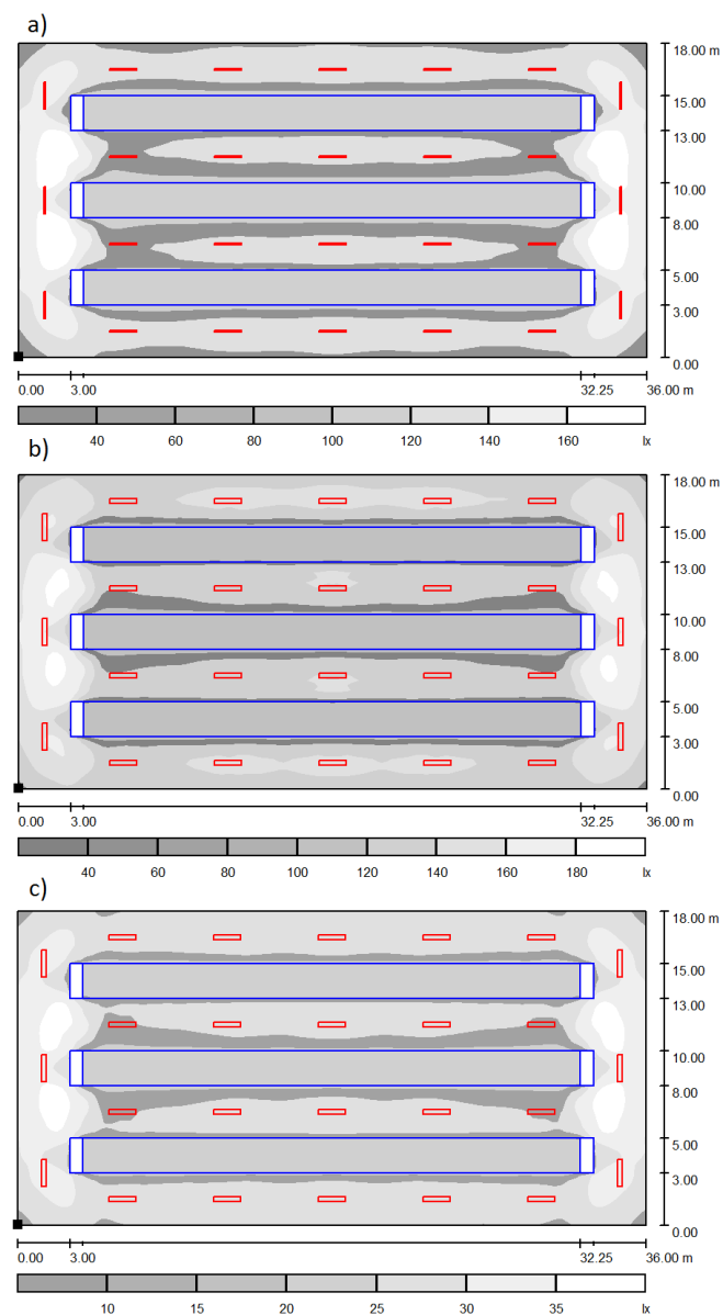
Rys. 5. Wyniki obliczeń natężenia oświetlenia przedstawione w stopniach szarości dla: a) oprawy LED, b) oprawy świetłówkowej do niskich temperatur, c) oprawy świetłówkowej tradycyjnej
