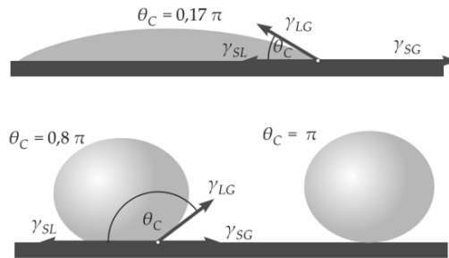
Fig. 1. Contact angle interpretation for good wetting, poor wetting, and no wetting [L. 1] Rys. 1. Kąt zwilżania dla dobrego zwilżania, słabego i całkowitego braku zwilżania [L. 1]
