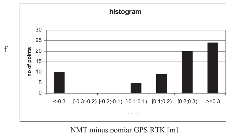
Rys. 8. Histogram rozkładu odchyłek pomiędzy NMT, a pomiarem GPS –RTK; 4 punkty o błędzie < -2.4 m; 12 punktów o błędzie w przedziale: [0.3 – 0.5 m), 9 w przedziale: [0.5 – 0.7) i 1 punkt o błędzie 1.3 m.
