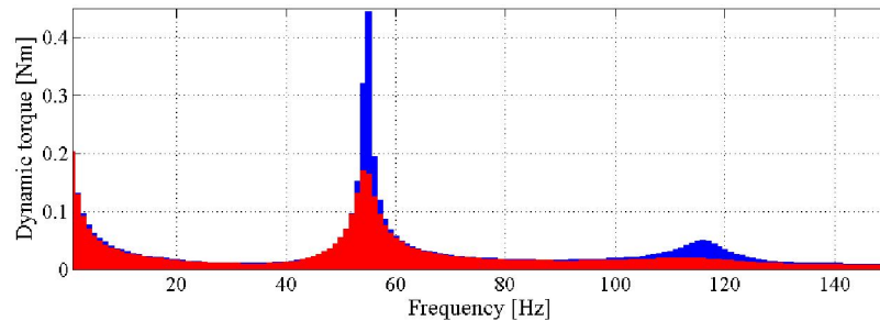
Rys. 3. Obliczone amplitudowe charakterystyki momentu dynamicznego (układ nietylniony- kolor niebieski, układ tłumiony- kolor czerwony)
