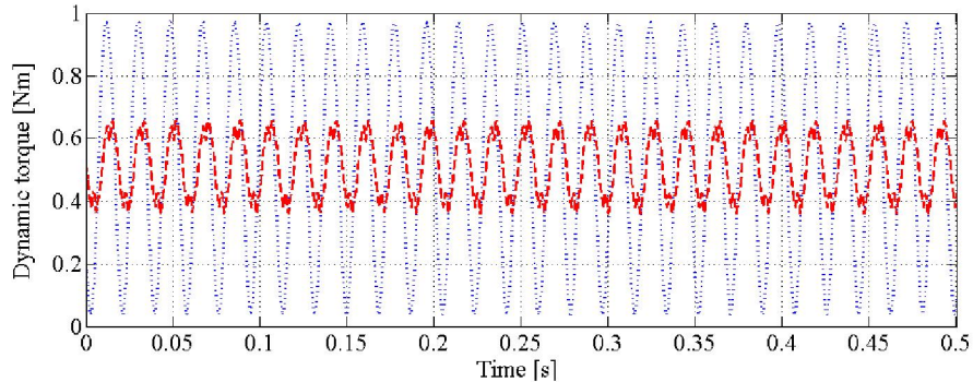
Rys. 2. Obliczony przebieg momentu dynamicznego (układ nietyumiony- kolor niebieski, układ tłumiony- kolor czerwony)
