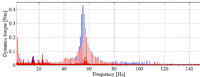
Rys. 5. Amplitudowe charakterystyki momentu dynamicznego zmierzone doświadczalnie (układ nietłumiony- kolor niebieski, układ tłumiony- kolor czerwony)
