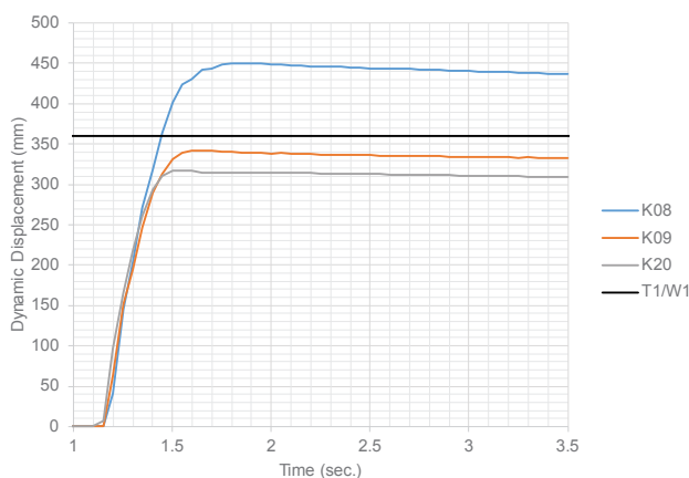
Rys. 6. Przemieszczenie boczne wybranych barier koncepcyjnych
