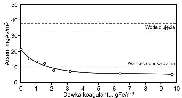
Rys. 1. Zawartość jonów arsenu w filtracie podczas oczyszczania wody podziemnej w procesie koagulacji powierzchniowej z zastosowaniem PIX 112 Fig. 1. Arsenic content in the filtrate during groundwater treatment by surface coagulation with PIX 112
