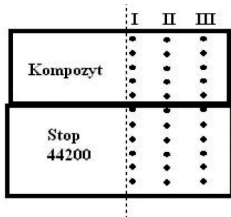
Rys. 12. Schemat pomiarów twardości w złączach stop 44200 - kompozyt.
