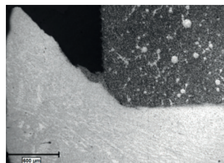
Rys. 15. Obrazy mikrostruktury złącza: stop-44200 + 30 % Al 2 O 3 .
