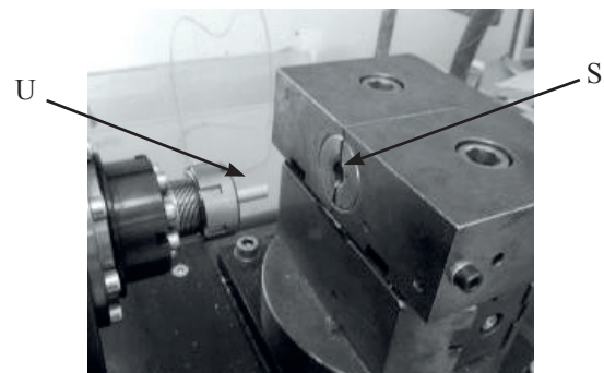
Rys. 7. Schemat procesu zgrzewania tarcowego: U - próbka ze stopu aluminium umieszczona w obrotowym wrzecionie, S - materiał kompozytowy umieszczony w nieruchomym uchwycie. Fig. 7. Scheme of friction welding process: U - Al alloy specimen mounted on rotary spindle, S - composite material in stationary clamp.
