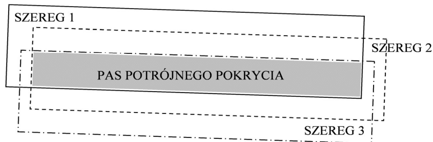
Rys. 1. Obszar potrójnego pokrycia dla zobrazowań ADS40
