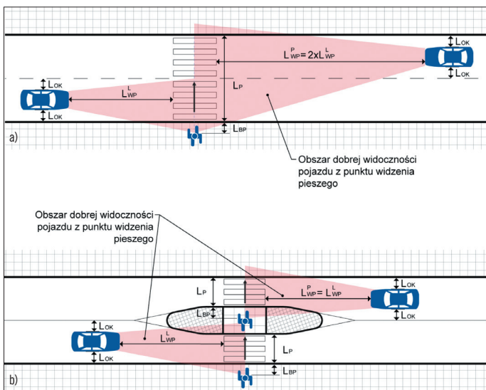
Rys. 4. Zasady wyznaczania obszaru dobrej widoczności na przejściach dla pieszych w Polsce: a) przejście przez jezdnię dwupasową, b) przejście przez jezdnię dwupasową z wyspą azylu.
