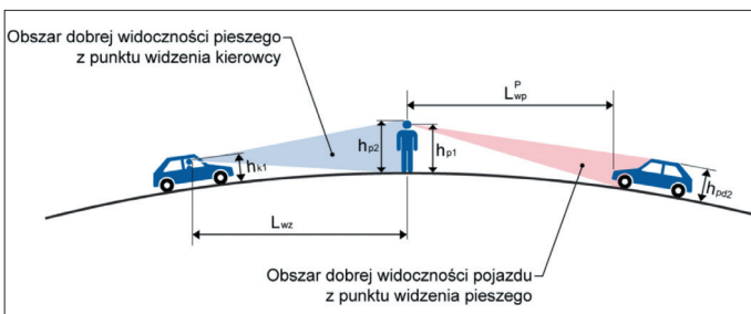
Rys. 6. Schemat sprawdzania warunków dobrej widoczności na przejściu dla pieszych w profilu podłużnym drogi.
