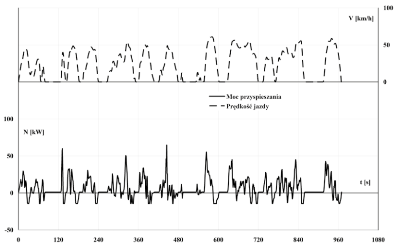
Rys. 15. Przebieg mocy prądu pobieranego z akumulatora dla jazdy realizowanej przez autopilota
