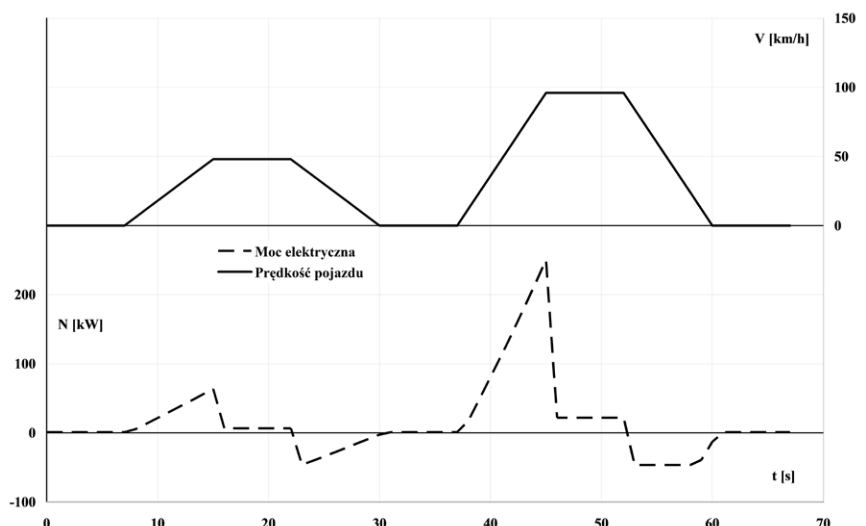
Rys. 4. Przebieg teoretyczny mocy elektrycznej oraz prędkości samochodu
