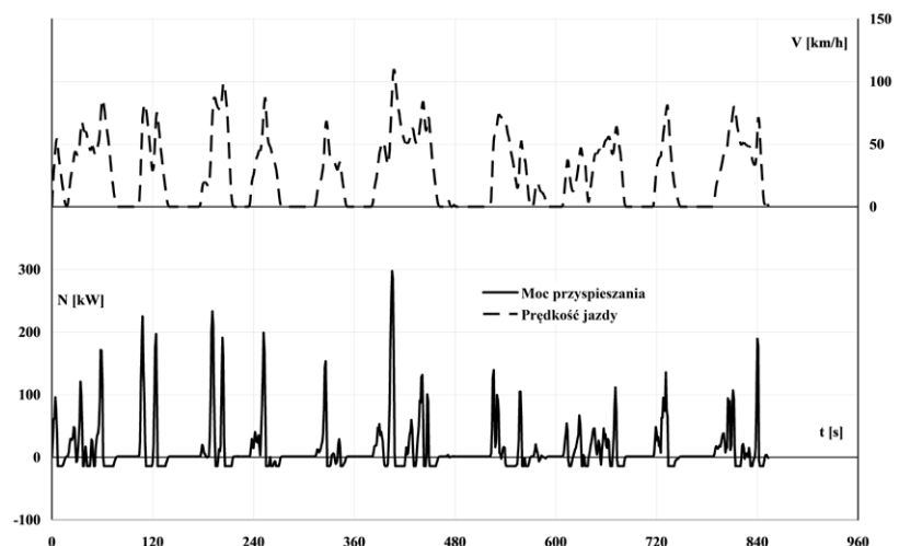
Rys. 14. Przebieg mocy prądu pobieranego z akumulatora dla dynamicznej jazdy realizowanej przez pierwszego kierowcę
