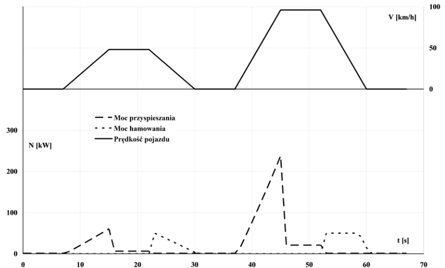
Rys. 3. Przebieg teoretyczny mocy potrzebnej do zmiany prędkości samochodu oraz prędkości samochodu
