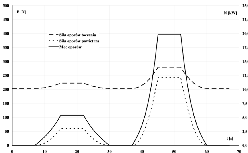
Rys. 2. Przebieg teoretyczny sił i mocy oporów
