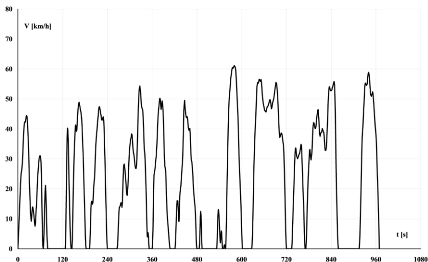
Rys. 6. Przebieg prędkości przy jeździe spokojnej
