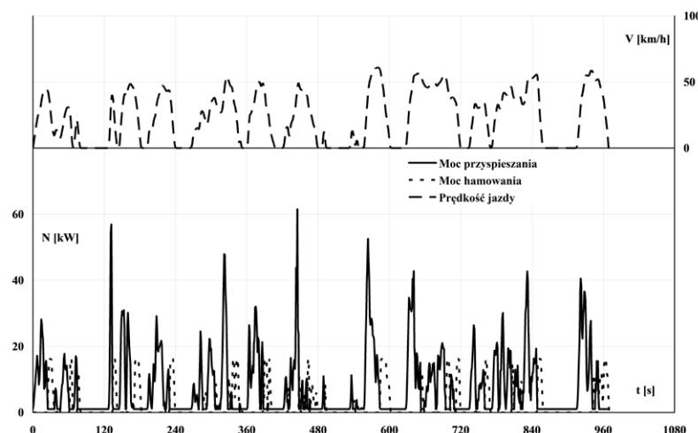
Rys. 10. Przebiegi mocy na kołach jezdnych i prędkości dla spokojnej jazdy realizowanej przez pierwszego kierowcę
