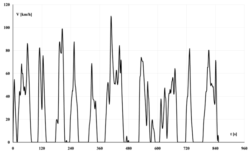
Rys. 7. Przebieg prędkości przy jeździe dynamicznej
