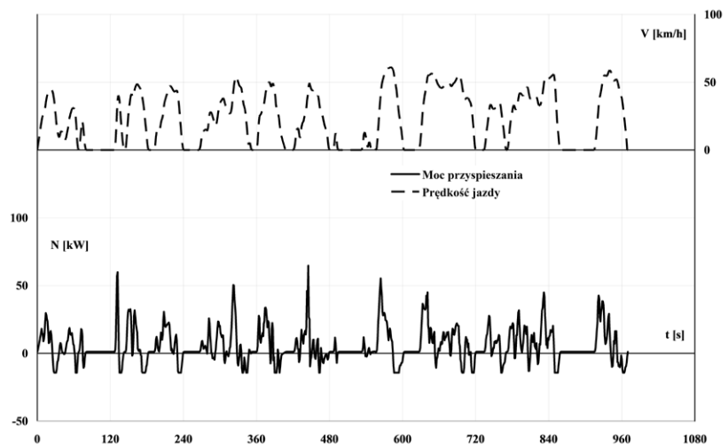
Rys. 13. Przebieg mocy prądu pobieranego z akumulatora dla spokojnej jazdy realizowanej przez pierwszego kierowcę
