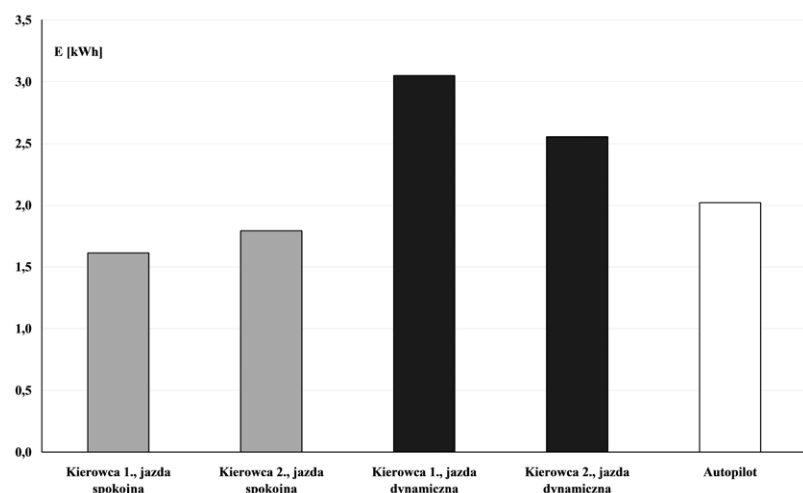
Rys. 9. Porównanie średniego zapotrzebowania na energię elektryczną
