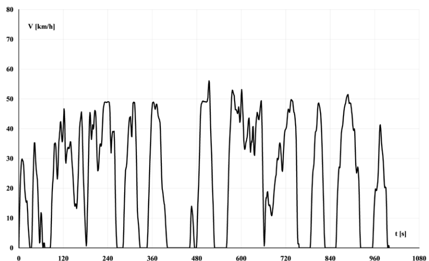
Rys. 8. Przebieg prędkości przy jeździe realizowanej przez autopilota
