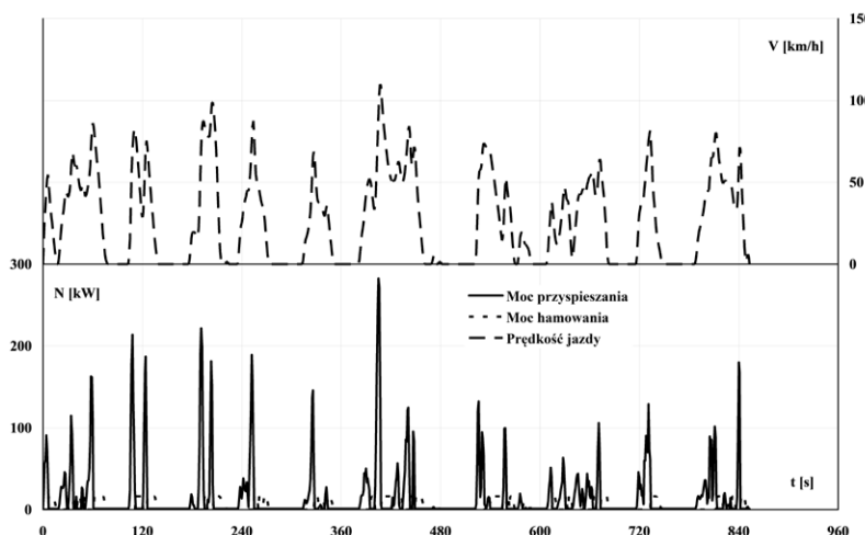
Rys. 11. Przebiegi mocy na kołach jezdnych i prędkości dla dynamicznej jazdy realizowanej przez pierwszego kierowcę
