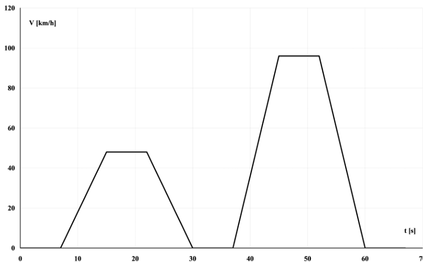
Rys. 1. Przebieg teoretyczny prędkości pojazdu
