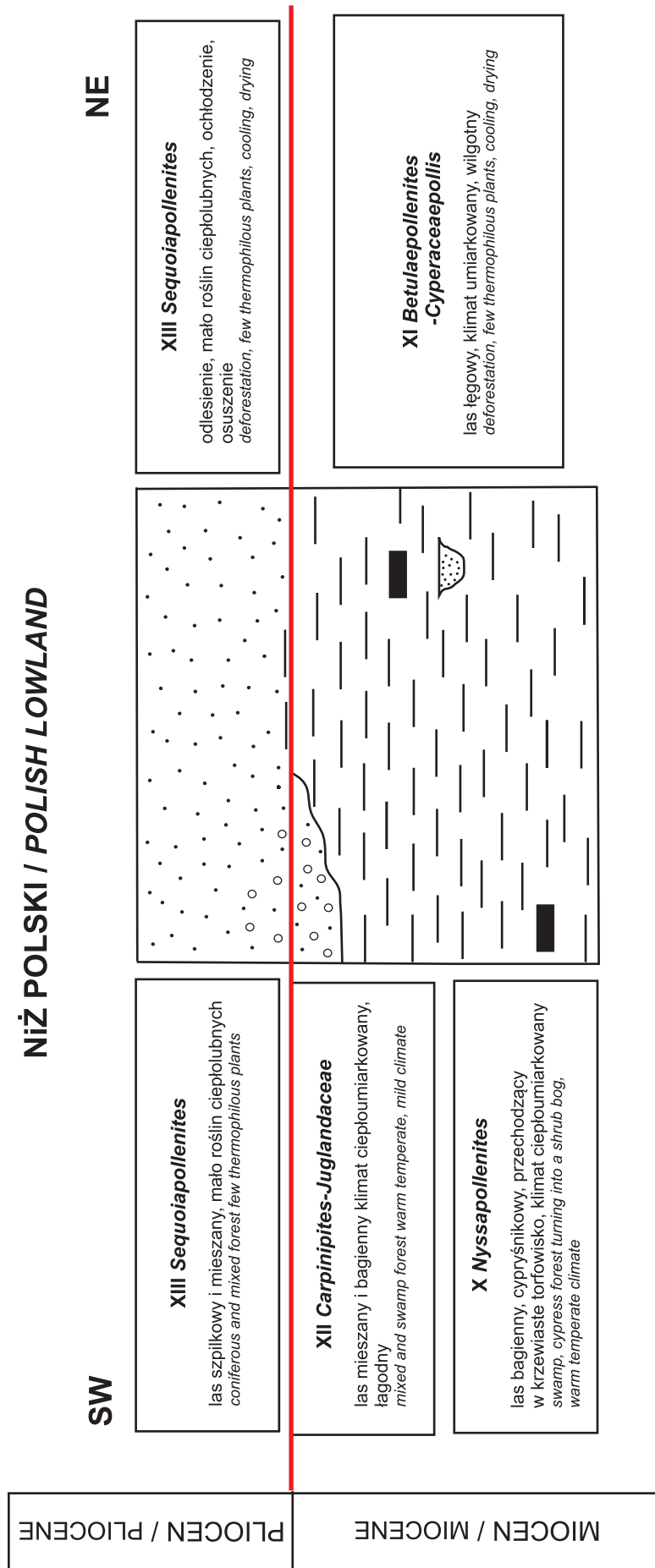
Fig. 7. Granica między miocenem górnym a pliocenem na Niżu Polskim
