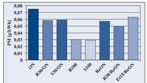
Rys. 3. Emisja cząstek stałych PM przy zasileniu paliwami konwencjonalnymi i biopaliwami [4]
