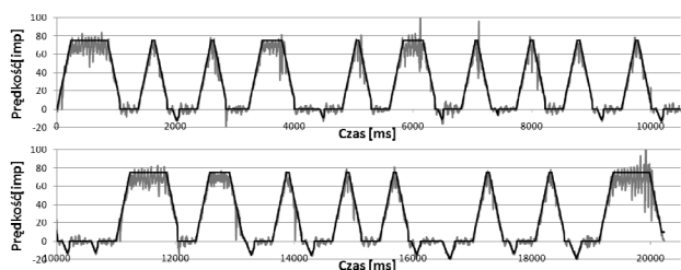
Rys. 18. Ruch liniowy robota wewnątrz drugiego labiryntu Fig. 18. Linear motion of the robot inside the second maze
