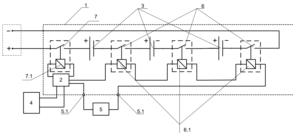
Rys. 1. Uproszczony schemat elektryczny połączenia modułów (3) baterii ze stycznikami (6) których uzwojenia sterujące (6.1) są połączone szeregowo i są połączone z akumulatorem niskonapięciowym (4), BMS (2) i czujnikiem uderzeniowym (5)
