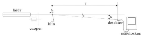
Rys. 5. Schemat układu eksperymentalnego do pomiaru współczynnika załamania światła
