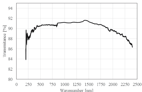
a. UV-VIS-NIR spectra of geopolymers PW/GEO
