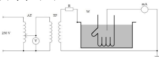
Rys. 1. Wysokonapięciowe stanowiska pomiarowego do badania sprzętu elektroizolacyjnego
