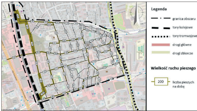
Rys. 17. Przykładowy obszar – kartogram natężeń ruchu pieszego
