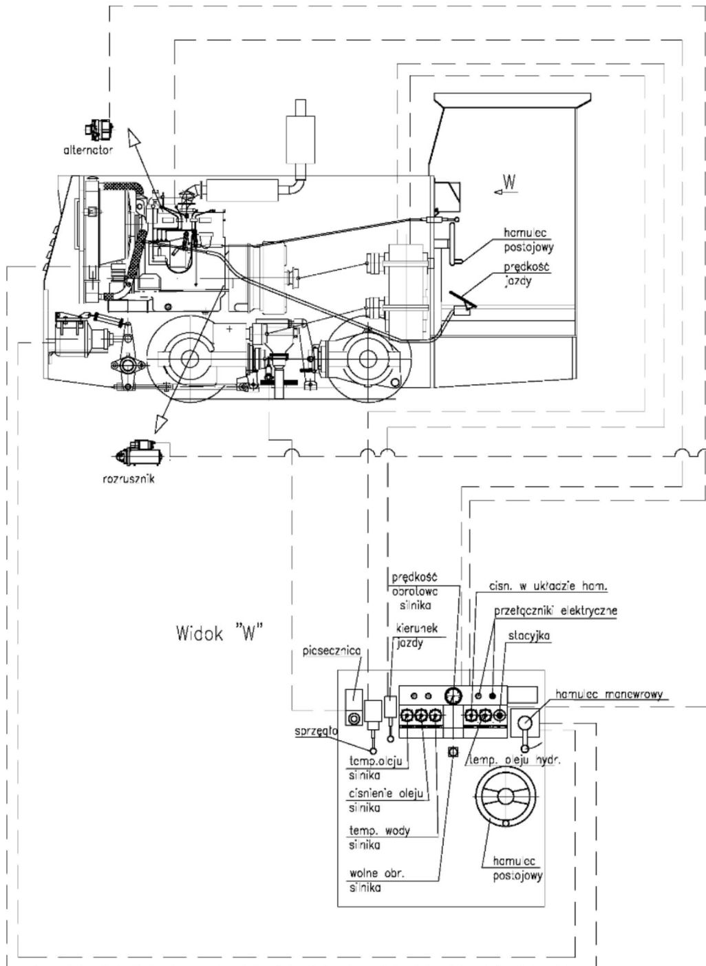
Rys. 5. Schemat sterowania mechanicznego lokomotywy WLP-85 oraz pulpitu sterowniczy [2]
