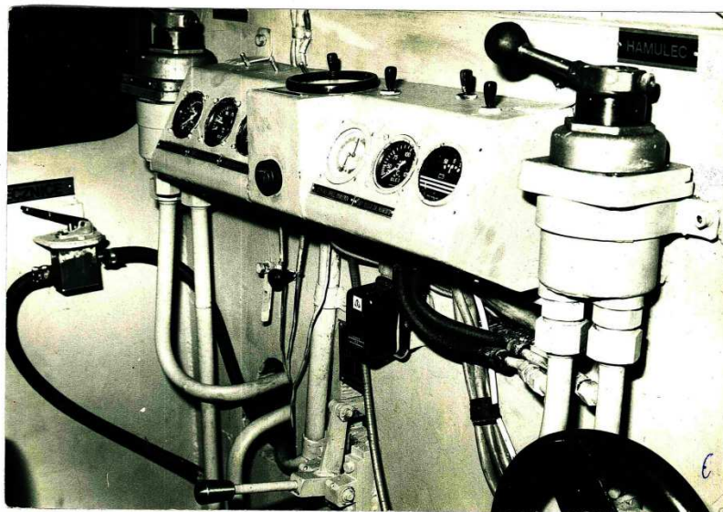
Rys. 4. Pulpit sterowniczy lokomotywy WLP-85 [7]
