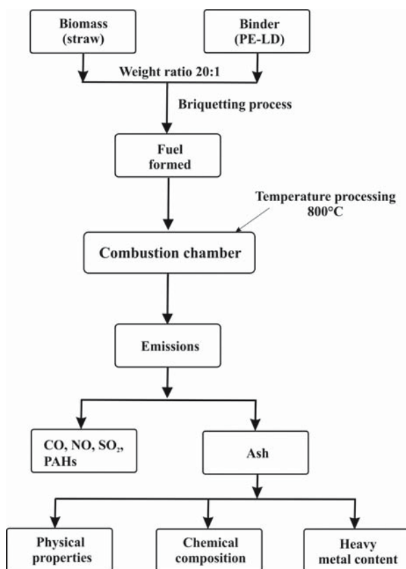
Fig. 2. Diagram of experiment (by M. Czop, M. Kajda-Szcześniak)
