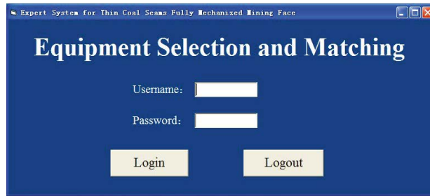
Fig. 4. Login interface
