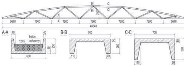
Rys. 2. Dźwigar o rozpiętości 48,84 m w magazynie na Nabrzeżu Rumuńskim w Gdyni
