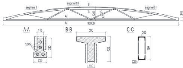
Rys. 8. Koncepcja dźwigara typu SDK na przykładzie elementu o rozpiętości 30 m
