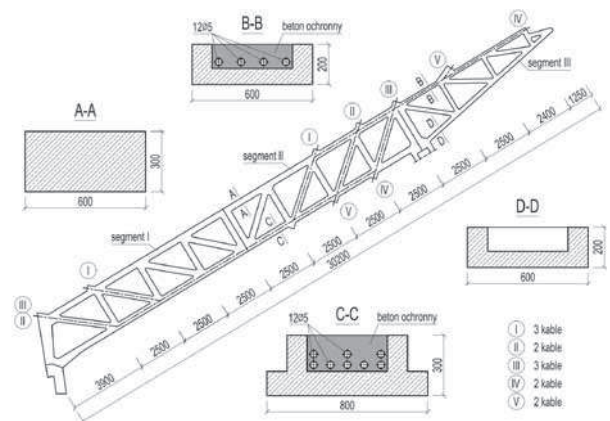
Rys. 11. Nietypowy dźwigar składany w konstrukcji stadionu
