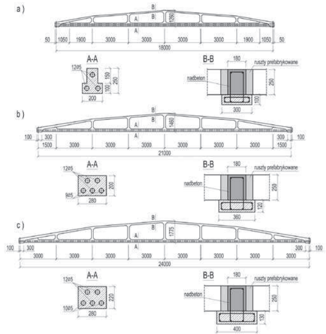
Rys. 1. Pierwsze dźwigary oszczędnościowe: a) KBO-18, b) KBO-21, c) KBO-24
