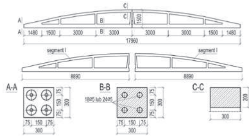
Rys. 9. Dźwigar KB-185
