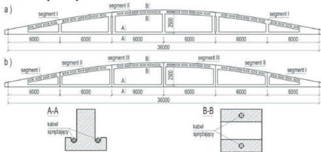
Rys. 7. Ogólna koncepcja elementów z „suchymi stykami”
