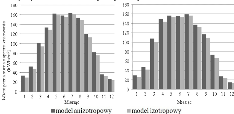
Rys.4-5. Miesięczne sumy napromieniowania na powierzchnię skierowaną na południe pochyloną pod kątem 45^\circ dla Warszawy (4) i Suwałki (5)
