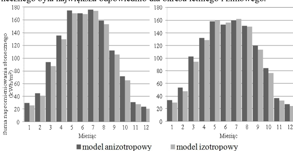
Rys.10-11. Miesięczne napromieniowanie na powierzchnię optymalnie zorientowaną dla modelu izotropowego i anizotropowego (po lewej stronie dla powierzchni optymalizowanej pod kątem maksymalizacji zysków słonecznych w okresie letnim) (po prawej stronie dla powierzchni optymalizowanej pod kątem maksymalizacji zysków słonecznych w okresie zimowym)
