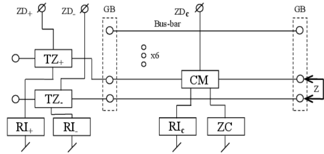
Rys. 1. Schemat blokowy części symulatora do testowania ciągłości połączeń oraz rezystancji izolacji, gdzie: GB – gniazda bananowe, ZD +/c – złącza diagnostyczne, Z – zwora, a także bloki symulujące: cewkę magnesu (CM), tor zasilania (TZ +/c ), rezystancję izolacji (RI +/c ) oraz zwarcia (ZC)
