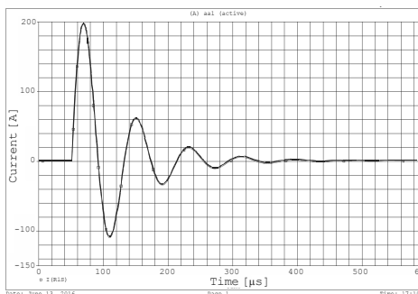
Rys. 6. Przebieg prądu dla C = 1,08 \mu F, L = 150 \mu F, R_{uz} = 115 \text{ m}\Omega oraz R_{fe} = 4 \Omega
