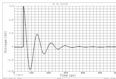
Rys. 5. Przebieg napięcia dla C = 1,08 \mu F, L = 150 \mu F, R_{uz} = 115 \text{ m}\Omega oraz R_{fe} = 4 \Omega
