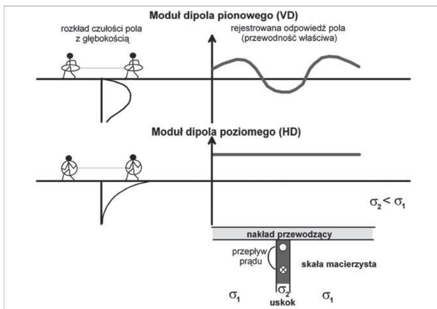
Rys. 5. Odpowiedź dla metody przewodności gruntu (przewodność pozorna, \sigma_a ) ponad przewodzącą dajką. Zasięg głębokości zmienia się z orientacją cewek [3] Fig. 5. Response of ground conductivity method (apparent conductivity, \sigma_a ) over conductive dike. The depth penetration changes along with coil orientation (McNeill 1997)
