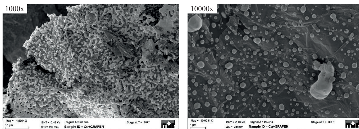
Fig. 2. SEM images of rGO covered with copper oxide, after annealing at 600°C. Rys. 2. Obrazy SEM rGO pokrytego tlenkiem miedzi, wyżarzzonego w temperaturze 600°C.
