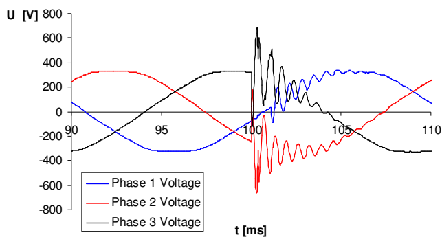
Rys. 5. Przepięcie wywołane załączeniem członu 20 kVAr baterii kondensatorów
