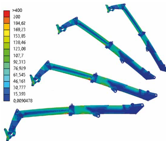
Rys. 13. Rozkład naprężeń w wysięgniku ładowarki obciążonym ładunkiem o wadze 1500 kg przy różnych kątach pochylenia wysięgnika
