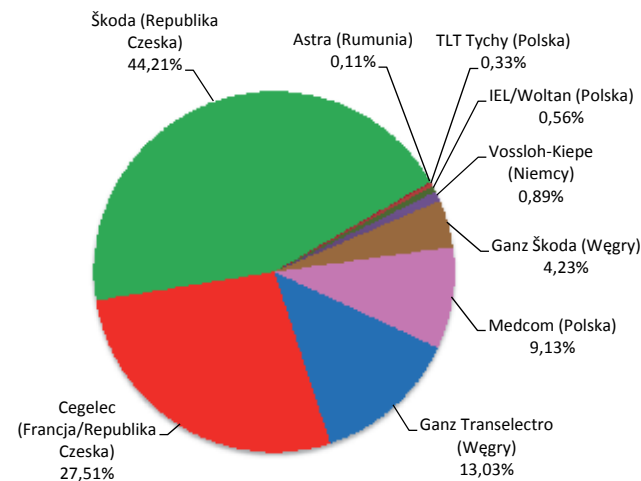
Rys. 2. Udział dostawców napędów w sumarycznej produkcji trolejbusów marki Solaris w latach 2001–2014
