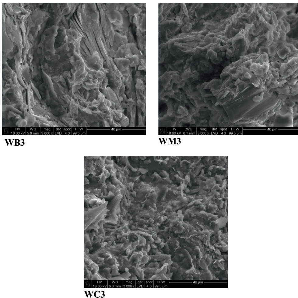
Rys. 7. Mikrofotografie SEM badanych surowców
