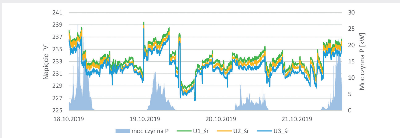
Rys. 2. Zmienność napięcia i mocy czynnej w funkcji czasu
