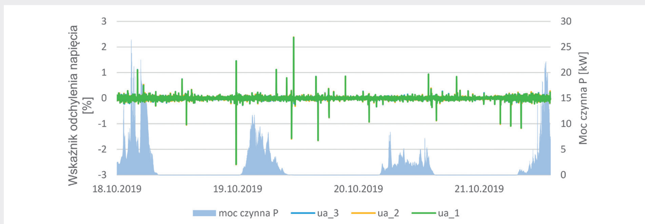
Rys. 3. Procentowy wskaźnik odchylenia napięcia oraz moc czynna w funkcji czasu
