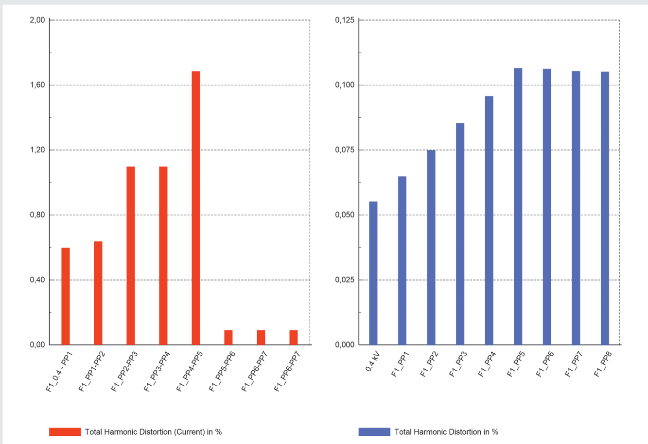
Rys. 7. Współczynnik THD prądu w liniach i THD napięcia na szynach obwodu z mikrogeneracją o P = 1,3 kW
