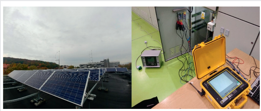
Fot. 1. Zdjęcia a) badanej instalacji fotowoltaicznej (z lewej) b) stanowiska pomiarowego (z prawej)
