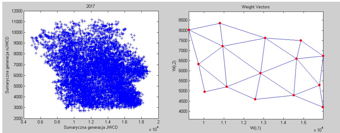
Figure 11. SOM neuron grids generated for the total generations of nJWCD and JWCD for 2017 data. Descriptions: Sumaryczna generacja JWCD (Pol.) - Total JWCD generation (Eng.), Sumaryczna generacja nJWCD (Pol.)- total nJWCD generation (Eng.). Source: Own elaboration in MATLAB and Simulink environment [6, 18, 20, 31].
