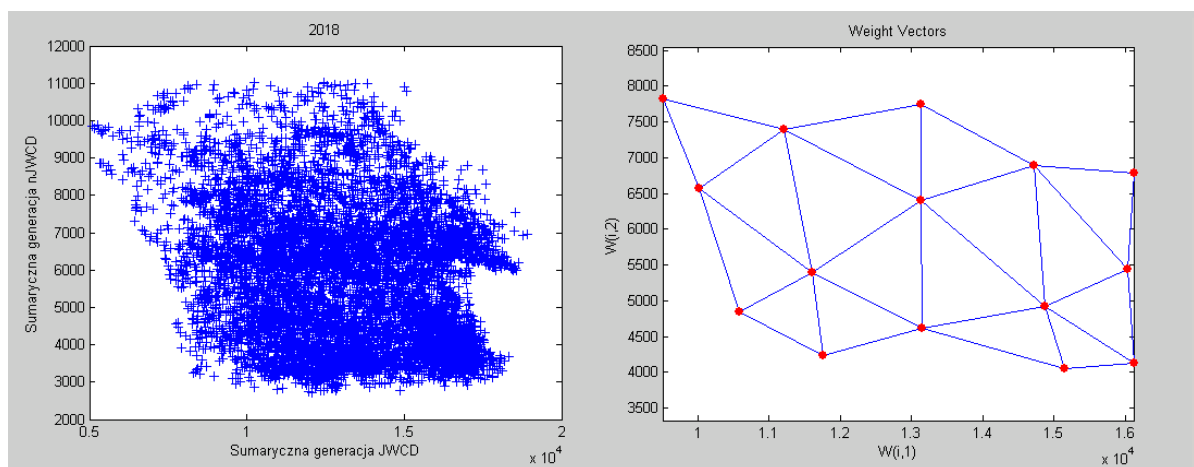
Figure 12. SOM neuron grids generated for the total generations of nJWCD and JWCD for 2018 data. Descriptions: Sumaryczna generacja JWCD (Pol.) - Total JWCD generation (Eng.), Sumaryczna generacja nJWCD (Pol.)- total nJWCD generation (Eng.). Source: Own elaboration in MATLAB and Simulink environment [6, 18, 20, 31].
