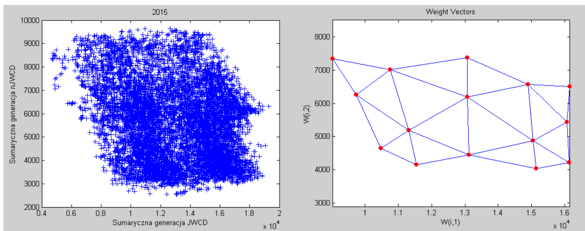
Figure 9. SOM neuron grids generated for the total generations of nJWCD and JWCD for 2015 data. Descriptions: Sumaryczna generacja JWCD (Pol.) - Total JWCD generation (Eng.), Sumaryczna generacja nJWCD (Pol.)- total nJWCD generation (Eng.). Source: Own elaboration in MATLAB and Simulink environment [6, 18, 20, 31].
