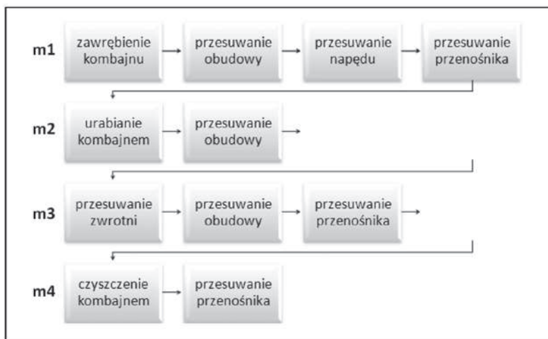
Rys. 2. Podział cyklu produkcyjnego realizowanego w przodkach ścianowych na moduły
