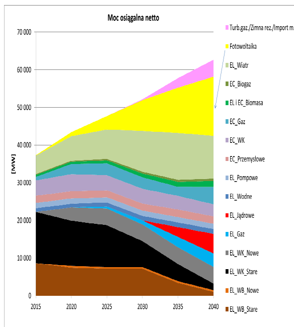
Rys. 1. Moc osiągalna netto źródeł wytwarzania energii elektrycznej wg zastosowanej technologii [2]
