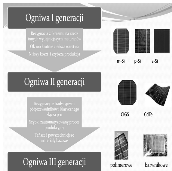
Rys. 3. Różne rodzaje ogniw fotowoltaicznych [10]
