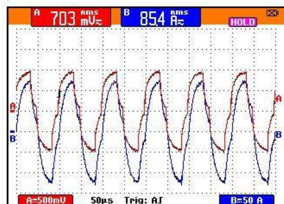
Rys. 7. Przebiegi napięciowo-prądowe w trakcie badań transformatora 30 kVA, 10 kHz w przypadku pełnego obciążenia: a) strona pierwotna, b) strona wtórna, skala napięcia 250V/dz
