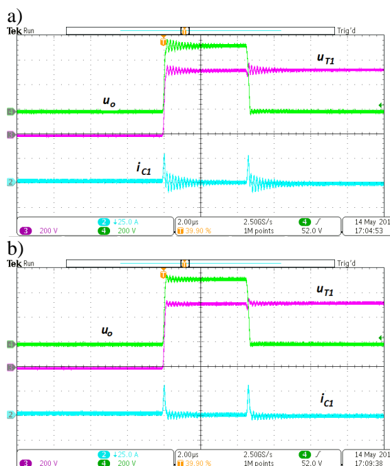
Rys. 4. Przebiegi prądu kondensatora i_{C1} , napięcia na tranzystorze T1 u_{T1} oraz napięcia na wyjściu ze stanowiska u_o w trakcie jednego cyklu przełączania F=20 kHz, a) t_{dead} = 1 \mu\text{s} , b) t_{dead} = 0,5 \mu\text{s}
