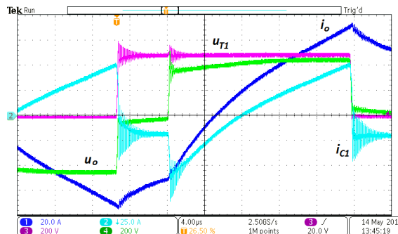
Rys. 3. Przebiegi prądu wyjściowego i_o , prądu kondensatora i_{C1} , napięcia na tranzystorze T1 u_{T1} oraz napięcia na wyjściu ze stanowiska u_o w trakcie jednego cyklu przełączania F=20 kHz
