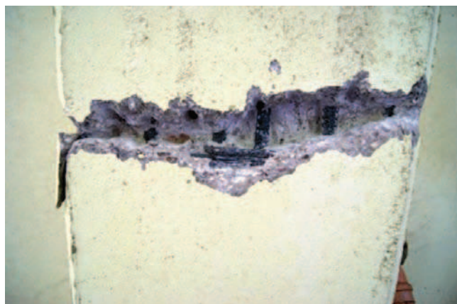
Rys. 1. Przykładowa odkrywka zbrojenia w poprzek całej szerokości belki
