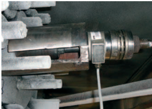
Rys. 7. Widok zainstalowanych elementów pomiarowych na głowicy zakotwienia czynnego
