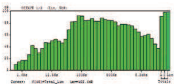
Rys. 5. Wartości poziomu ciśnienia akustycznego w funkcji częstotliwości dla nagłośnienia typu „głośna muzyka”
