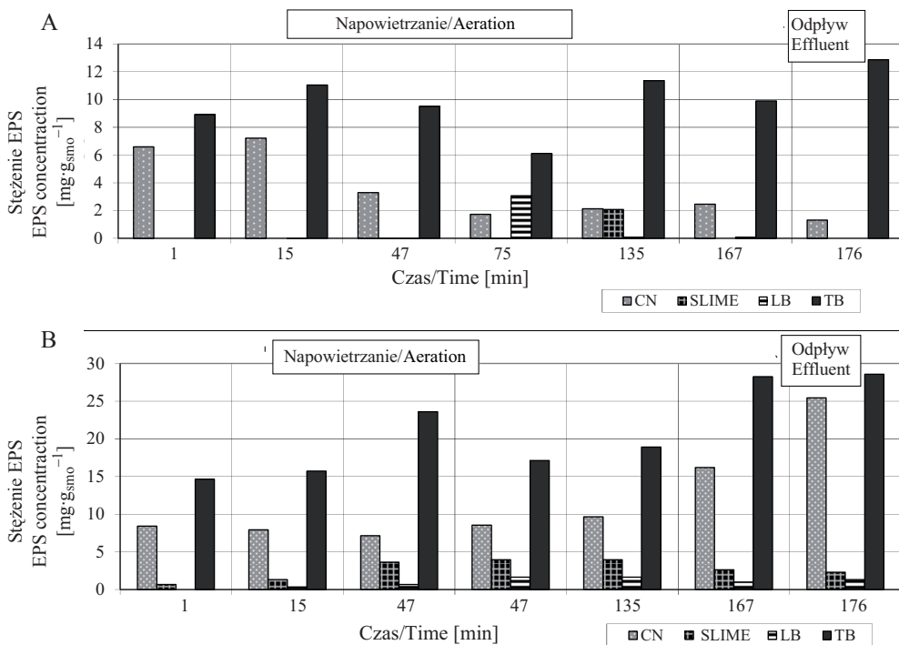
RYСУNEK 3. Zmiana zawartości zewnątrzkomórkowych białek (A) i polisacharydów (B) w różnych frakcjach EPS podczas jednego cyklu pracy reaktora (60. doba). Oznaczenia w tekście
