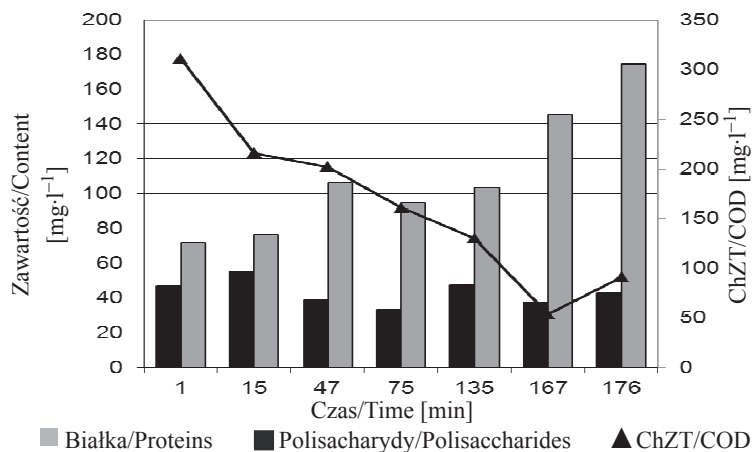
RYСУNEK 2. Zmiany zawartości białek, polisacharydów i ChZT w czasie jednego cyklu w 60. dobie prowadzenia eksperymentu
