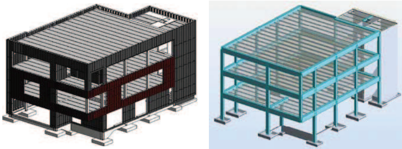
Rys. 3. Model geometryczny i analityczny konstrukcji w ramach projektu [11]
