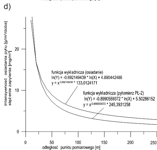
Rys. 3. Ekstrapolacja wyników stężenia pyłu i jego osiadania pyłu w strefie zabezpieczającej: a) chodnik wentylacyjny ściany I, b) przekop badawczy, c) chodnik wentylacyjny ściany II, d) pochylnia badawcza
