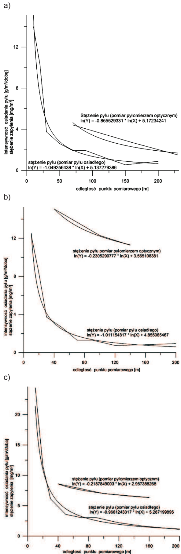
Rys. 1. Wyniki pomiarów stężenia pyłu w powietrzu i jego osiadania w strefie zabezpieczającej: a) chodnik wentylacyjny ściany I, b) przekop badawczy, c) chodnik wentylacyjny ściany II, d) pochylnia badawcza
