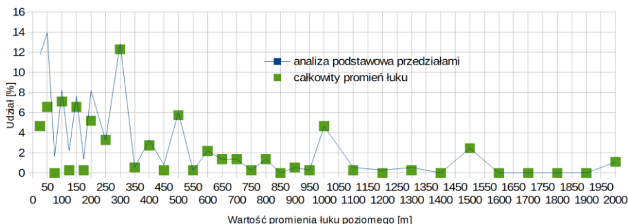
Rys. 4. Udział procentowy zinwentaryzowanych wartości promieni łuków tramwajowych w Gdańsku
