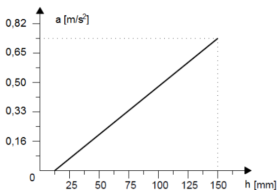
Rys. 3. Zalecana zależność pomiędzy przyspieszeniem nie zrównoważonym a przechyłką (na podstawie [35])
